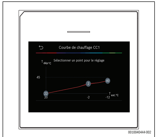
Fig. 1 Écran de démarrage pour le réglage de la courbe de chauffage pour le type de régulation de la température extérieure avec pied de courbe (et point de confort)
