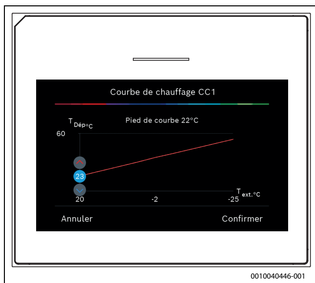
Fig. 3 Régler le pied de courbe (uniquement si le type de réglage est défini sur la température extérieure avec pied de courbe)
