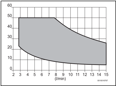
Fig. 30 Modèle 15 litres
