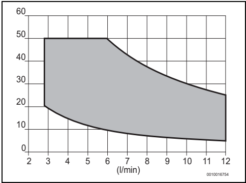
Fig. 29 Modèle 12 litres
