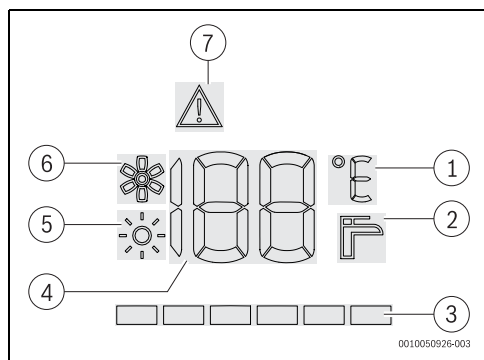
Fig. 5 Ecran
