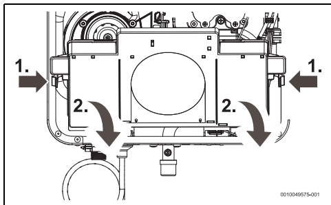
Fig. 24 Inclinaison du module de commande
