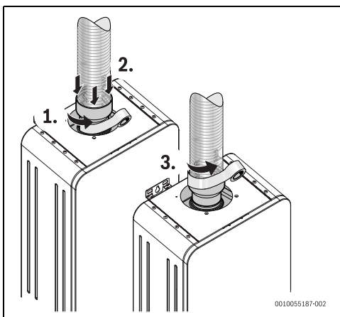
Fig. 22 Installation du type B23
