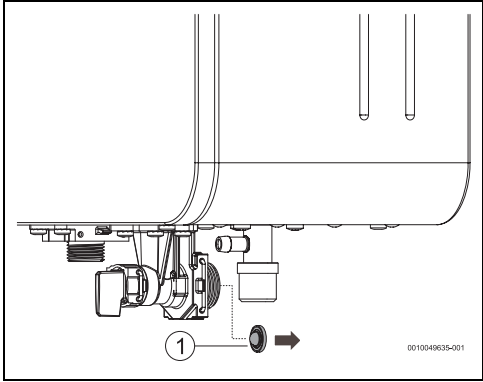
Fig. 27 Filtre à eau
