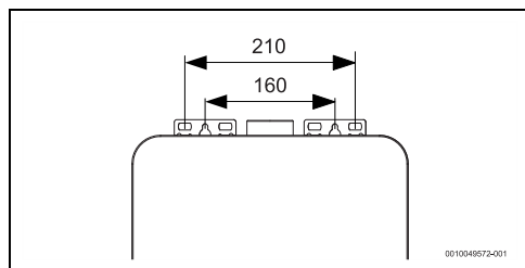
Fig. 19 Points de fixation
