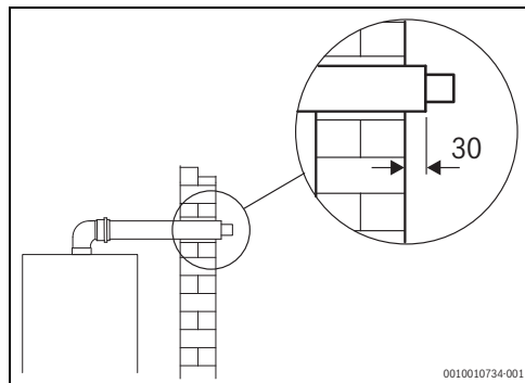
Fig. 23 Dimensions (en mm)
