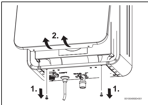
Fig. 26 Démontage de l'habillage avant
