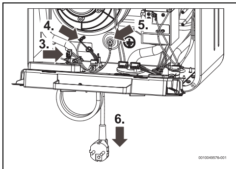
Fig. 25 Raccordements du câble de réseau
