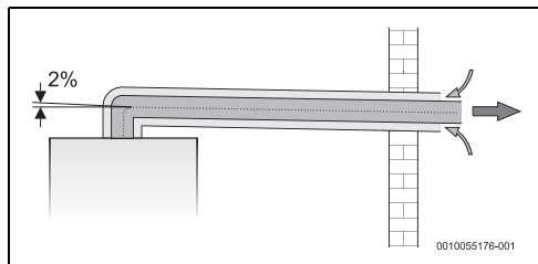
Fig. 21 Installation du type C13
