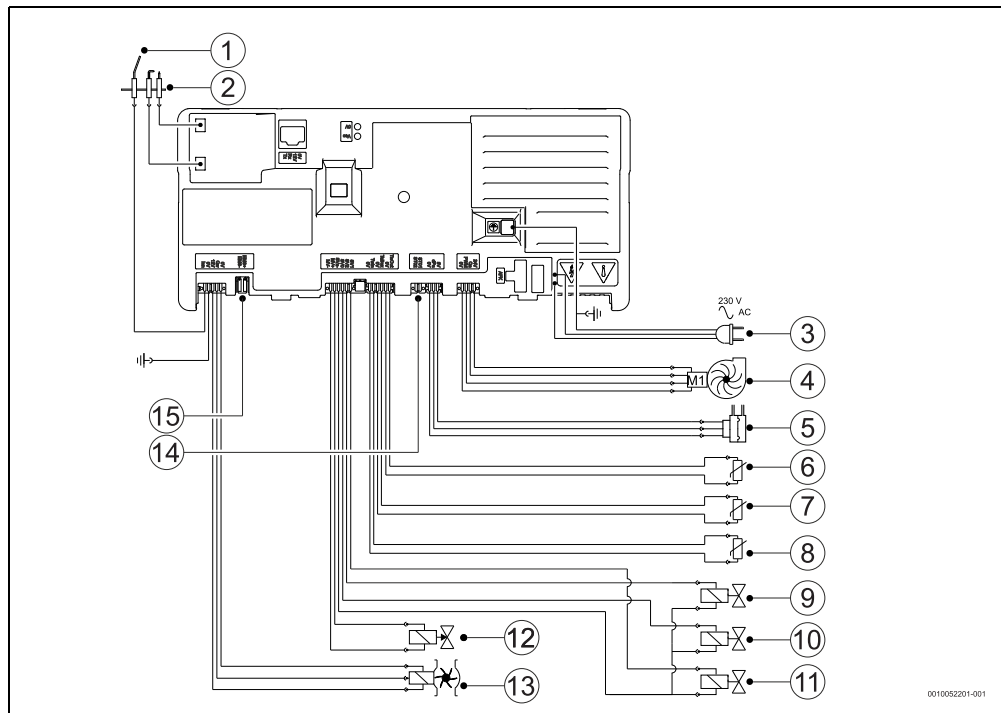
Fig. 28 Schéma de connexion
