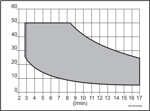
Fig. 31 Modèle 17 litres
