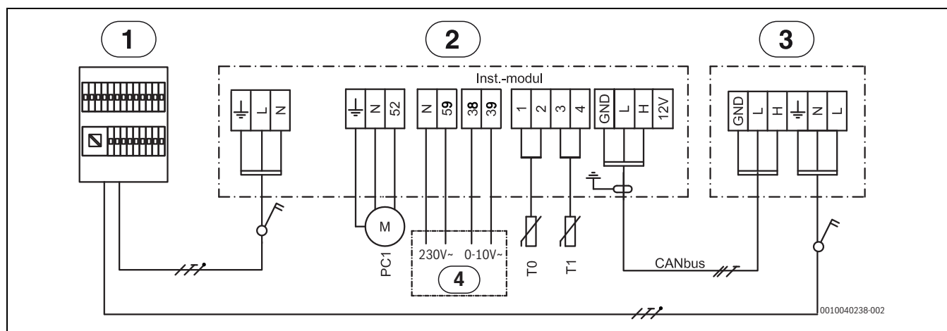
Afb. 42 Elektrisch schema
