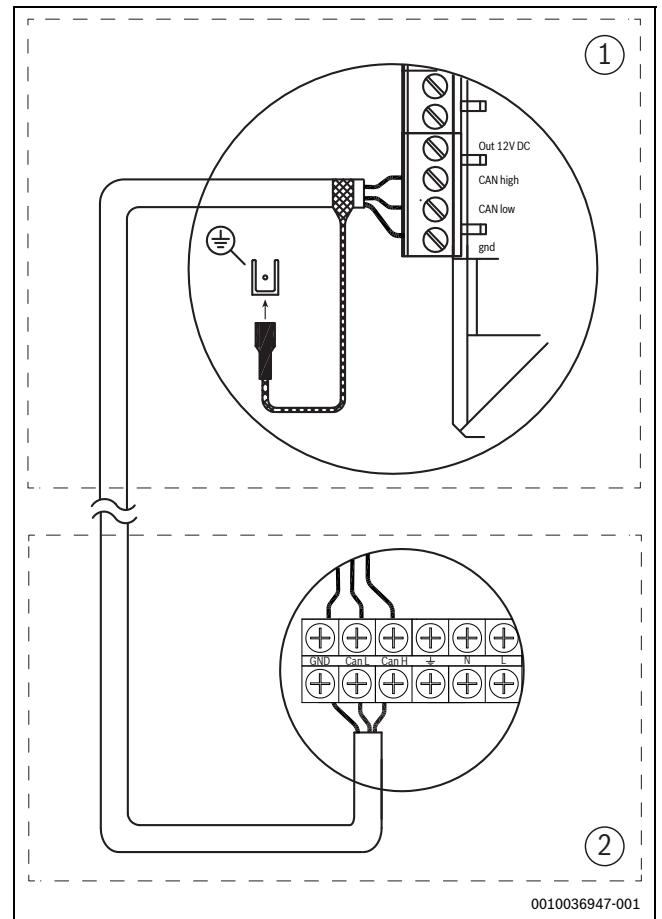
Afb. 12 CAN-BUS-aansluiting
