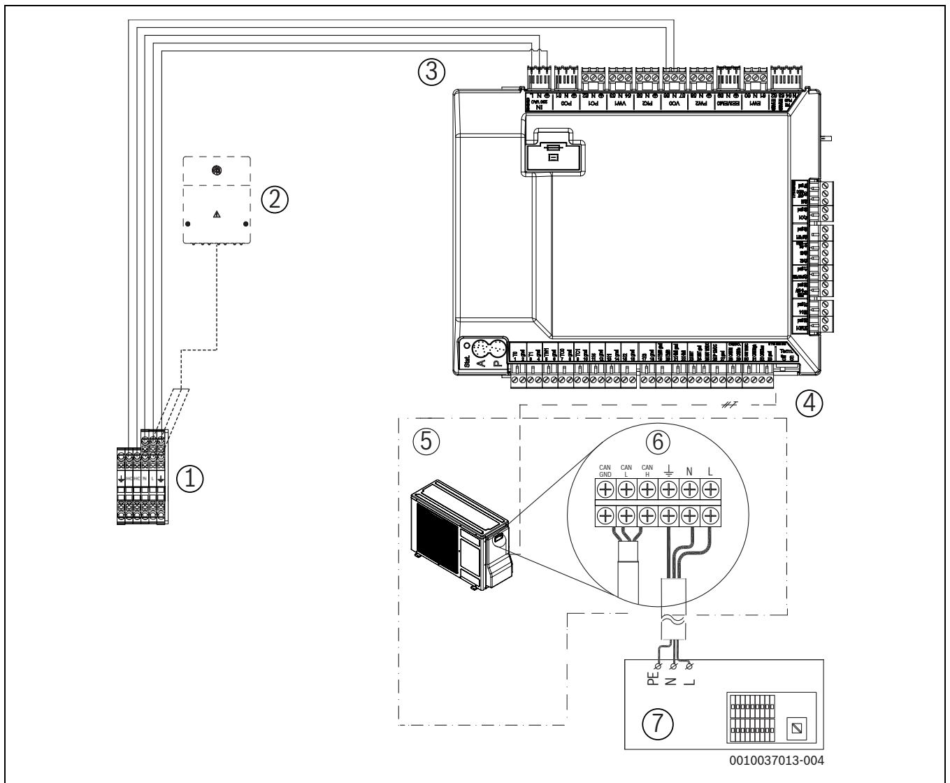
Afb. 43 Binneneenheid met 230 V~ buiteneenheid
