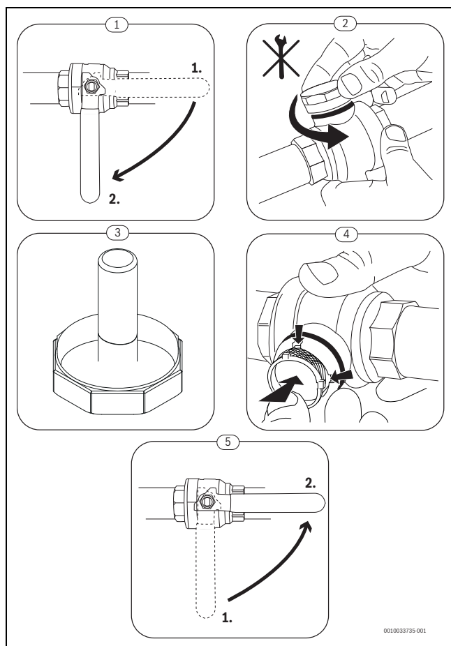
Afb. 19 Deeltjesfilter reinigen
