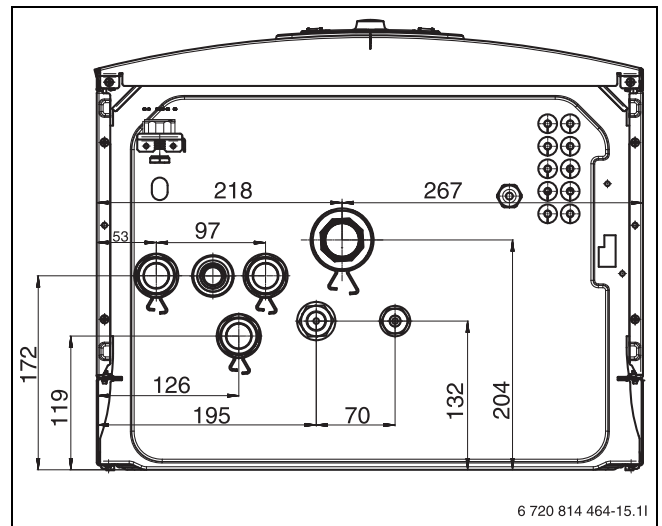
Afb. 5 Afmetingen en aansluitingen (aanzicht zonder lekbak)
