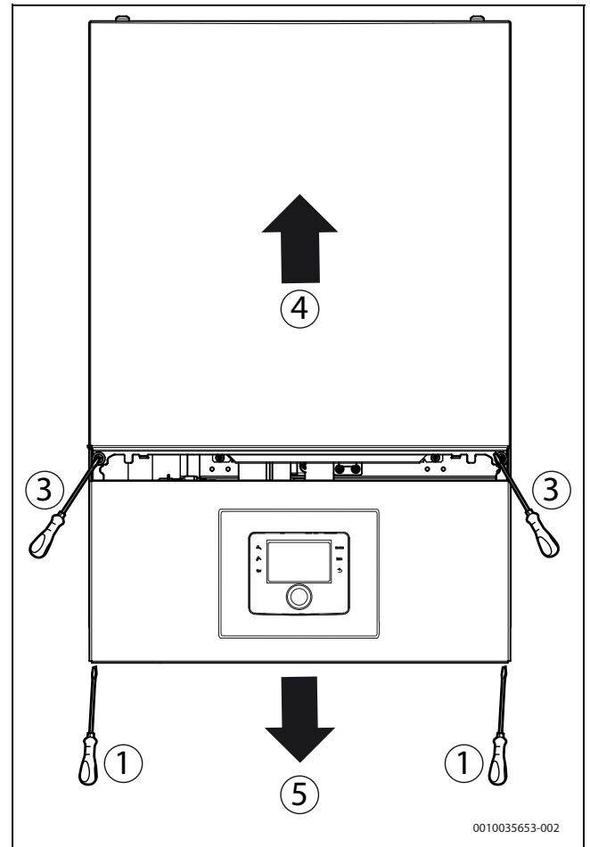
Afb. 6 Verwijder frontpaneel
