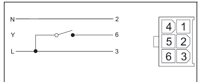
Afb. 23 Molex-stekker
