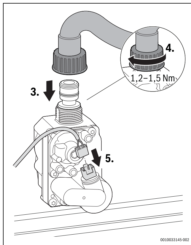
Fig. 62 Raccordement du tuyau du gaz et du connecteur – Respect du couple de serrage
