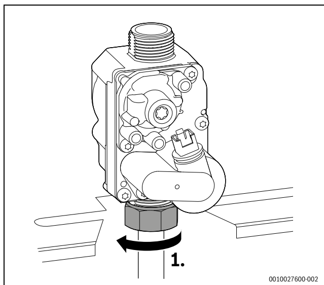
Fig. 57 Desserrage de l'écrou
