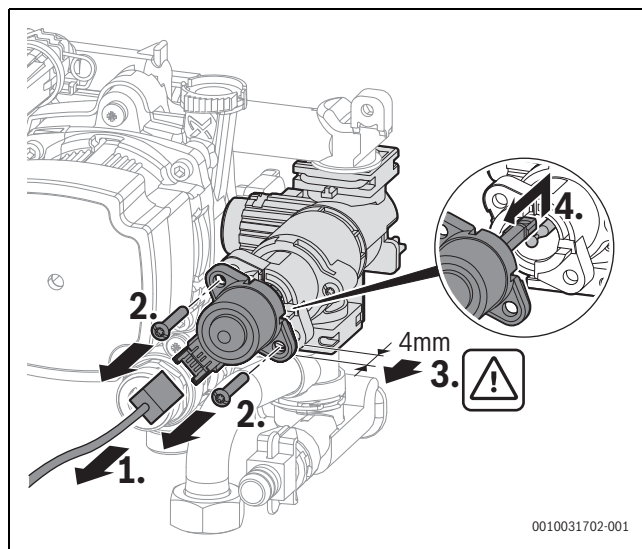
Fig. 71 Démontez le moteur au niveau de la vanne sélective (variante avec vis)
