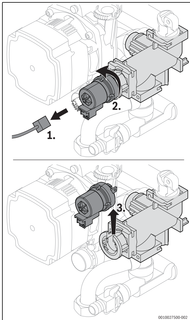
Fig. 69 Démontez le moteur au niveau de la vanne sélective (variante sans vis)
