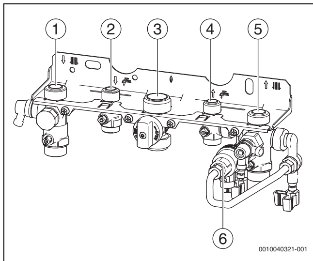
Fig. 37 Raccordements côté gaz et eau
