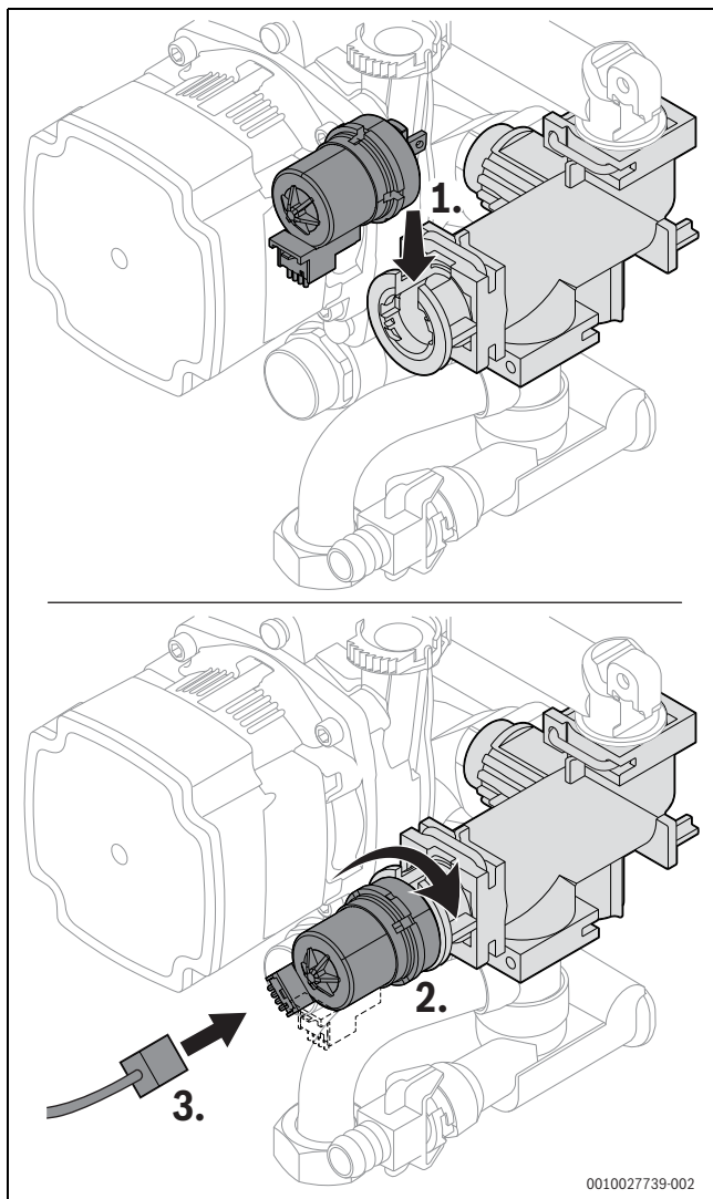
Fig. 70 Remonter le moteur au niveau de la vanne sélective (variante sans vis)
