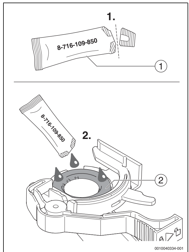
Fig. 67 Graisser le joint
