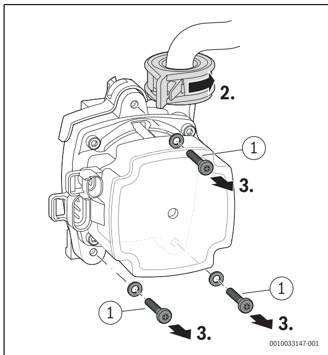
Fig. 52 Déverrouiller la pompe de chaudière et retirer les vis
