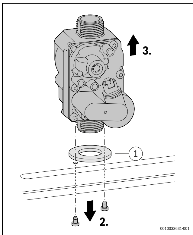
Fig. 58 Démontage du bloc gaz
