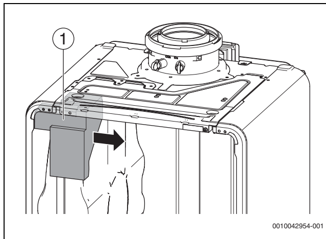
Fig. 32 Retirer la mousse de support
