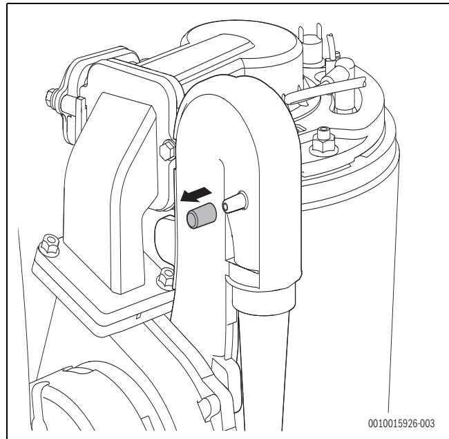
Fig. 49 Tubulure de mesure sur le dispositif de mélange
