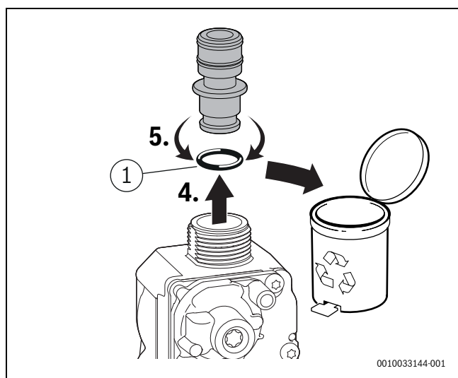
Fig. 56 Retrait de l'orifice
