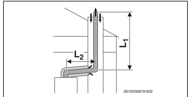
Fig. 17 Evacuation des fumées rigide selon C 93x dans le conduit et circuit d'air et de fumées concentrique dans le local d'installation
