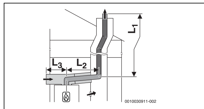
Fig. 15 Conduite d'évacuation des fumées flexible selon C 53x dans le conduit et circuit d'air et de fumées avec alimentation d'air séparée et conduite d'évacuation des fumées concentrique dans le local d'installation
