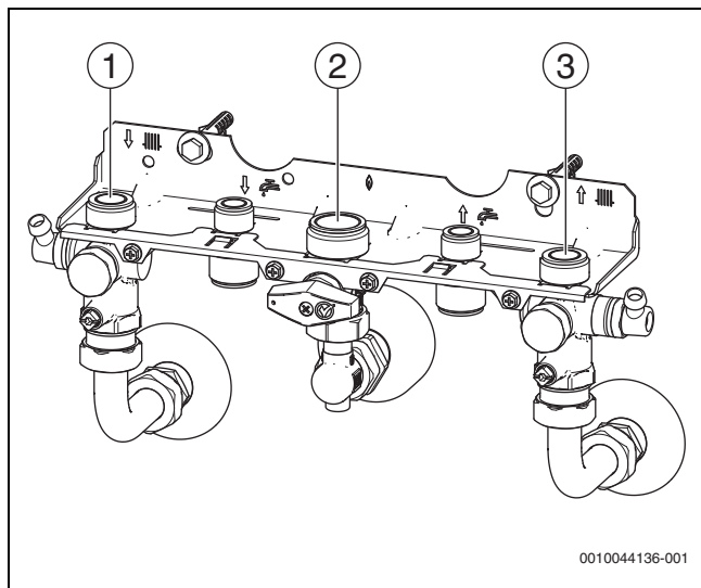
Fig. 38 Raccordements côté gaz et eau
