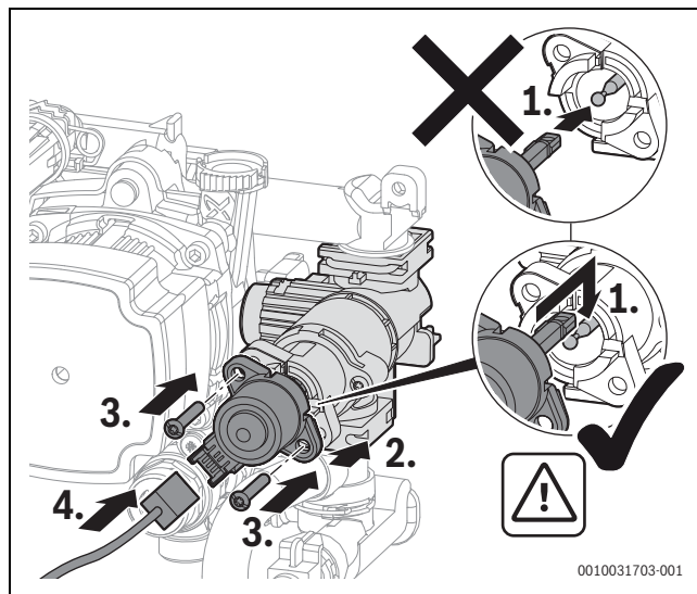
Fig. 72 Remonter le moteur au niveau de la vanne sélective (variante avec vis)
