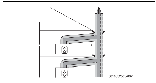
Fig. 24 Raccordement de plusieurs foyers selon C (12)3x avec circuit d'air et de fumées concentrique dans le local d'installation
