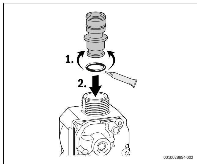
Fig. 61 Insertion l'orifice de réglage de gaz
