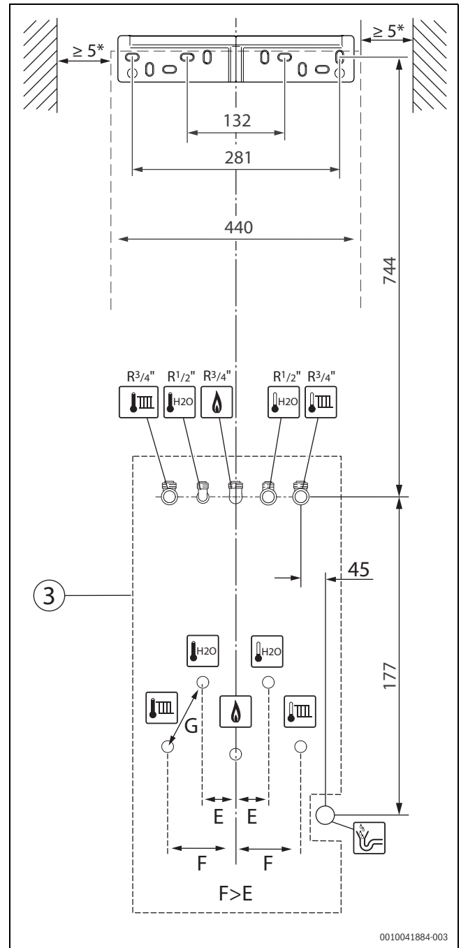
Fig. 5 Vue avant (mm)
