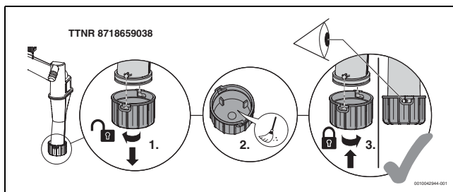
Fig. 65 Nettoyer le filtre.
