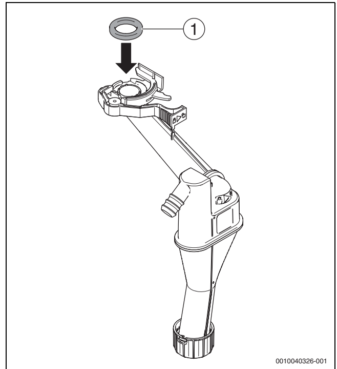
Fig. 66 Mise en place du nouveau joint sur le siphon de condensats
