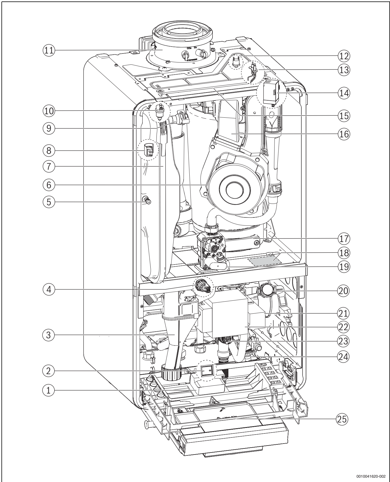
Fig. 7 Aperçu produit Accumulateur
