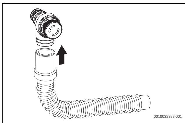
Fig. 33 Montage du tube sur la soupape de sécurité (chauffage)
