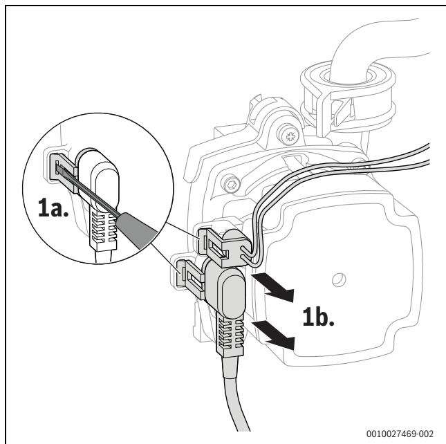
Fig. 51 Débrancher le connecteur de la pompe de chaudière
