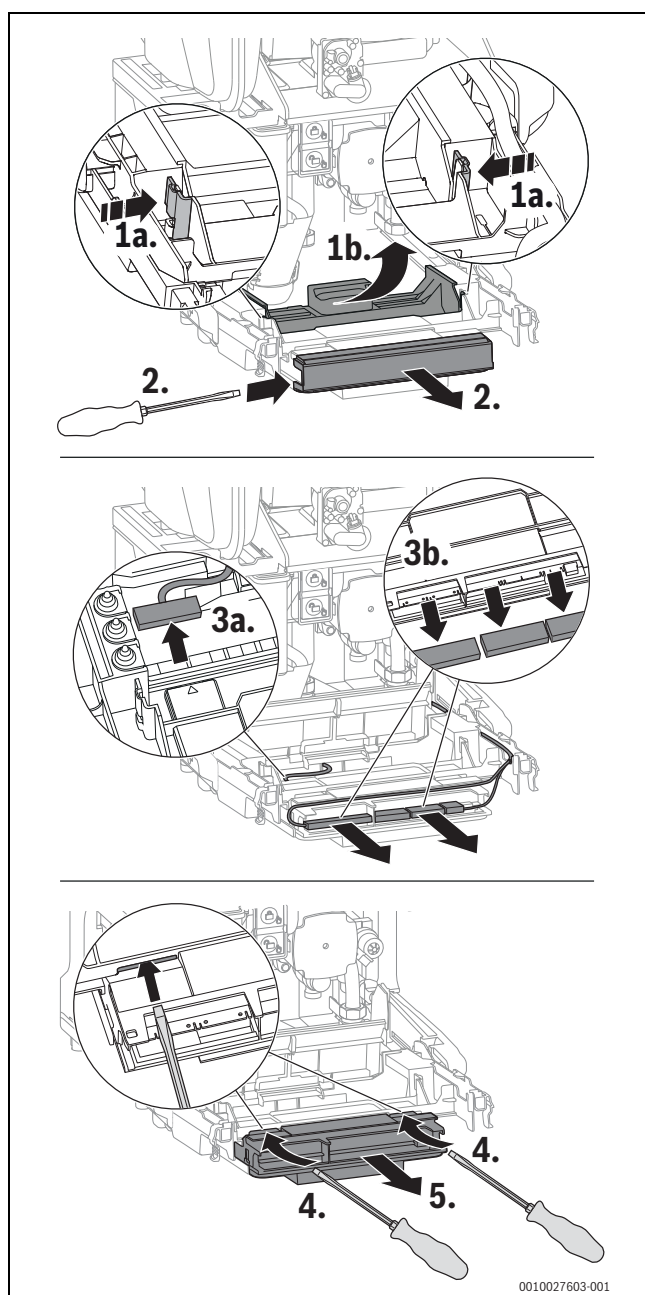
Fig. 63 Retirer l'appareil de commande
