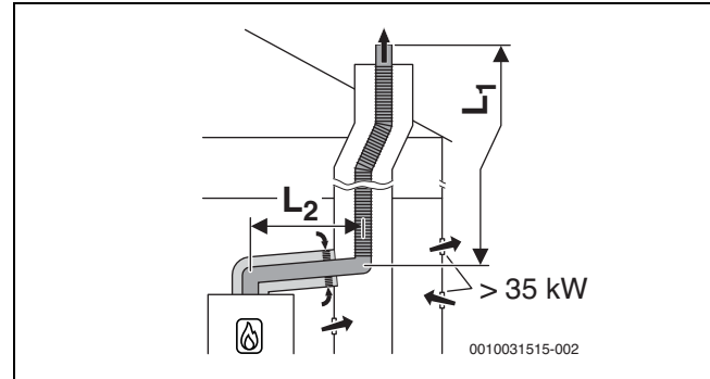
Fig. 22 Evacuation des fumées flexible dans le conduit selon B 33 avec arrivée d'air dépendant de l'air ambiant par le circuit d'air et de fumées concentrique dans le local d'installation
