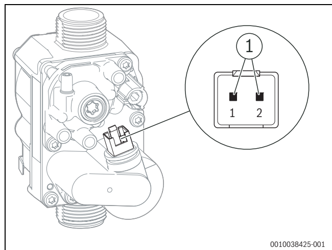
Fig. 50 Points de mesure du bloc gaz
