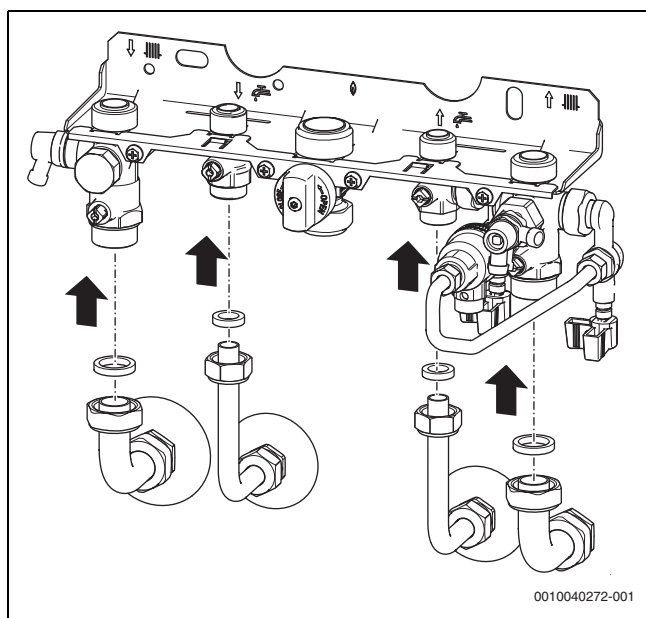
Fig. 31 Monter les tubes avec les joints sur la plaque de montage pour le raccordement (accessoire)
