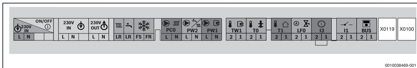
Fig. 41 Bornier pour accessoires externes
