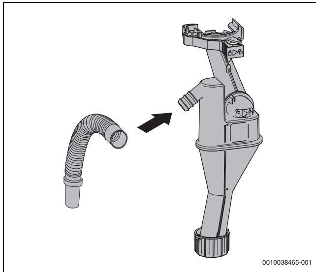
Fig. 34 Placer l'évacuation des condensats sur le raccord
