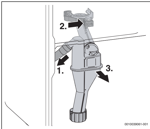
Fig. 64 Démontez le siphon des condensats
