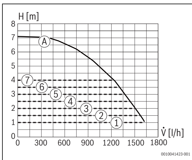
Fig. 73 Diagrammes de pompe et courbes caractéristiques de pompe
