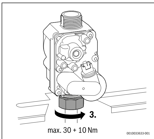
Fig. 60 Respect du couple de serrage
