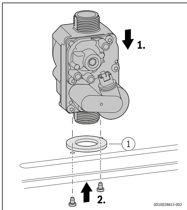
Fig. 59 Installation du bloc gaz
