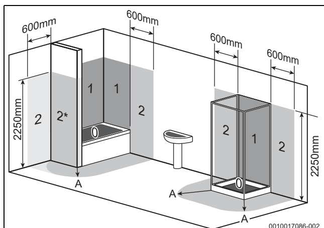
Fig. 29 Volumes de protection (exemple)
