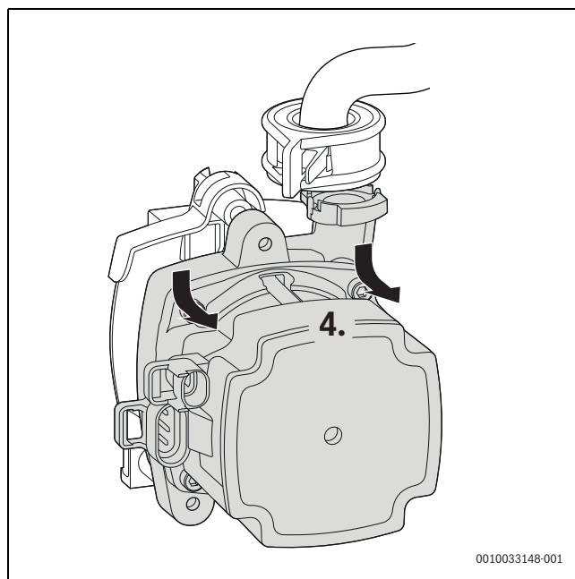
Fig. 53 Retirer la pompe de chaudière par l'avant
