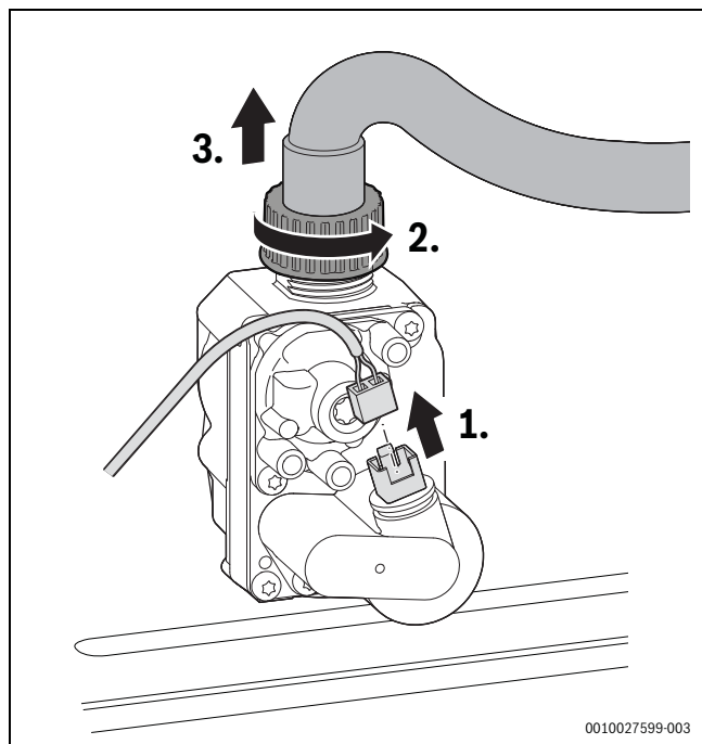
Fig. 55 Retrait du connecteur du bloc gaz et de l'écrou avec le tuyau du gaz
