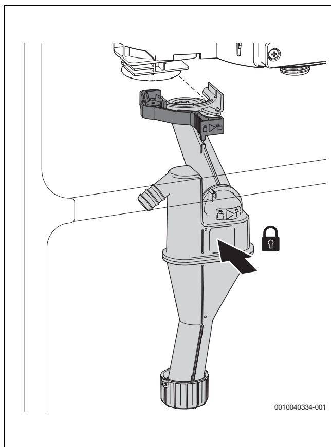
Fig. 68 Insertion du siphon de condensats
