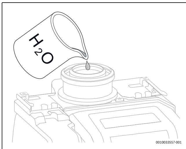
Fig. 35 Remplir le siphon des condensats avec de l'eau
