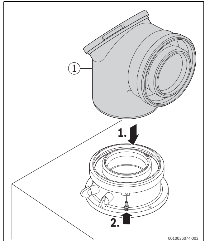
Fig. 36 Insérer les accessoires de fumisterie et fixer avec une vis.
