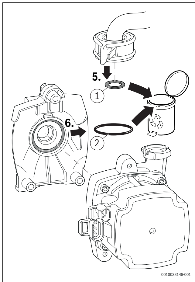
Fig. 54 Éliminer les joints
