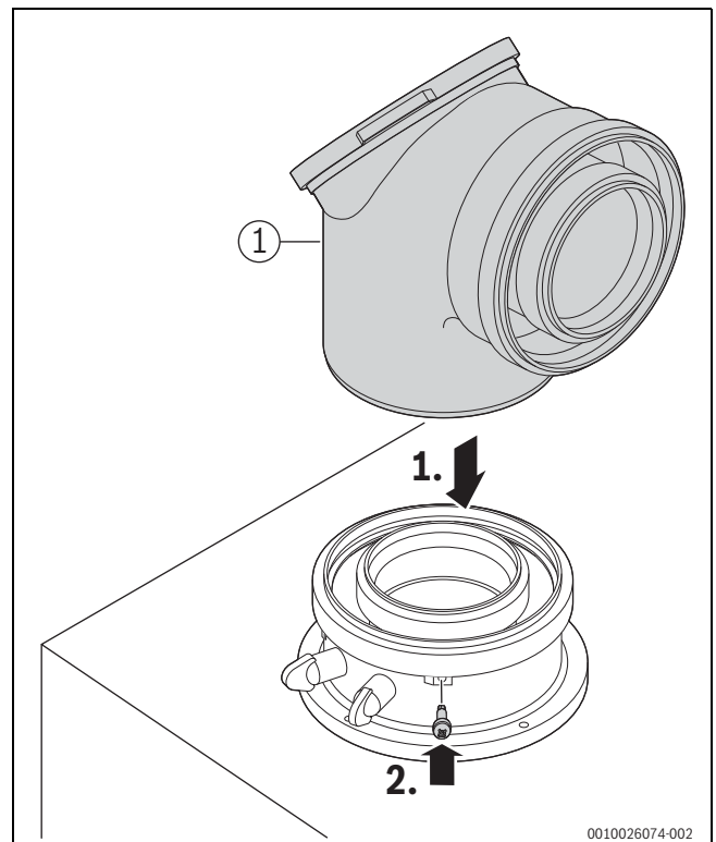
Bild 36 Abgaszubehör einsetzen und mit Schraube sichern
