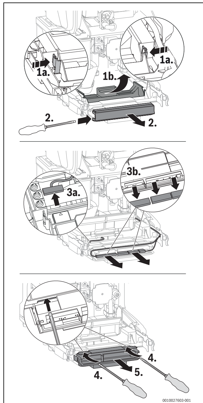
Bild 63 Steuergerät herausnehmen
