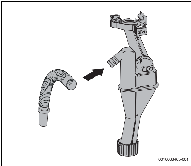
Bild 34 Kondensatablauf auf das Anschlussstück stecken
