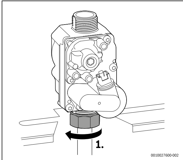
Bild 57 Überwurfmutter lösen
