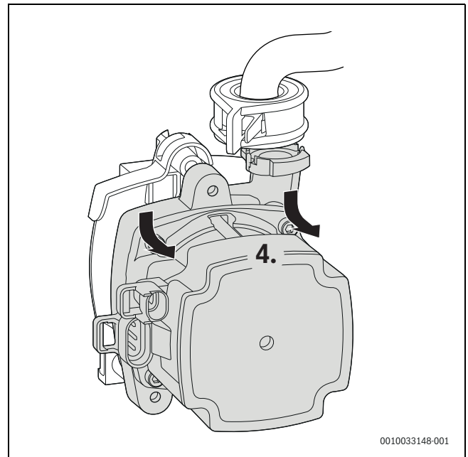
Bild 53 Heizungspumpe abnehmen
