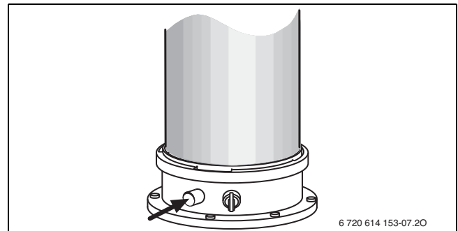
Bild 45 Abgasmessstutzen
