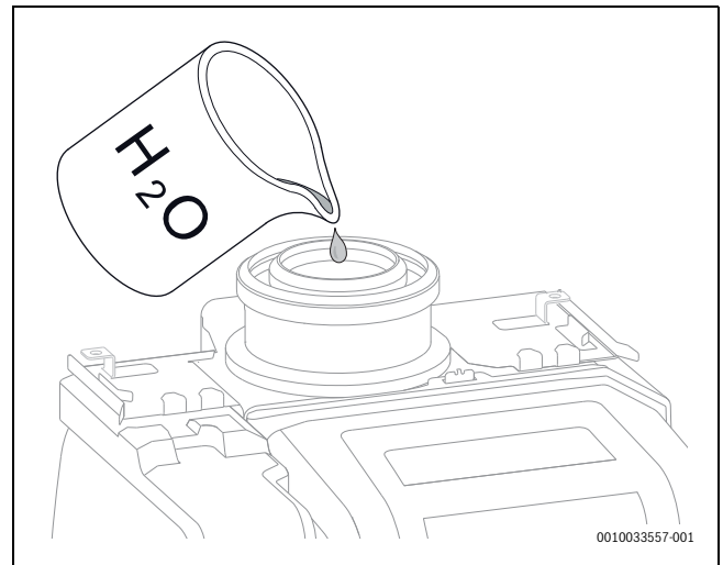
Bild 35 Kondensatsiphon mit Wasser füllen
