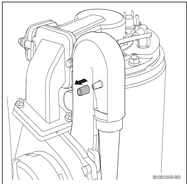
Bild 49 Messstutzen an der Mischeinrichtung
