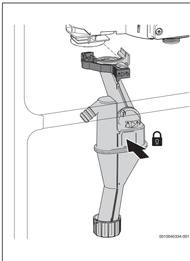
Bild 68 Kondensatsiphon einsetzen
