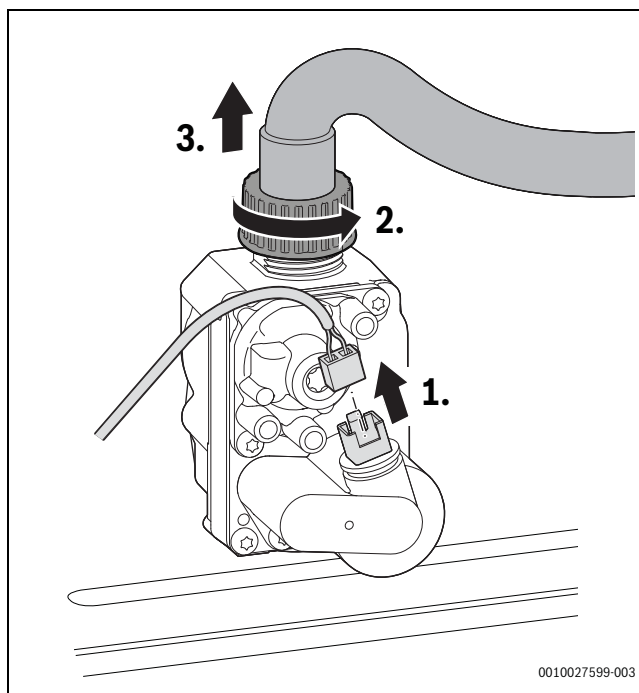
Bild 55 Stecker an der Gasarmatur abziehen und Überwurfmutter mit Gasschlauch abnehmen
