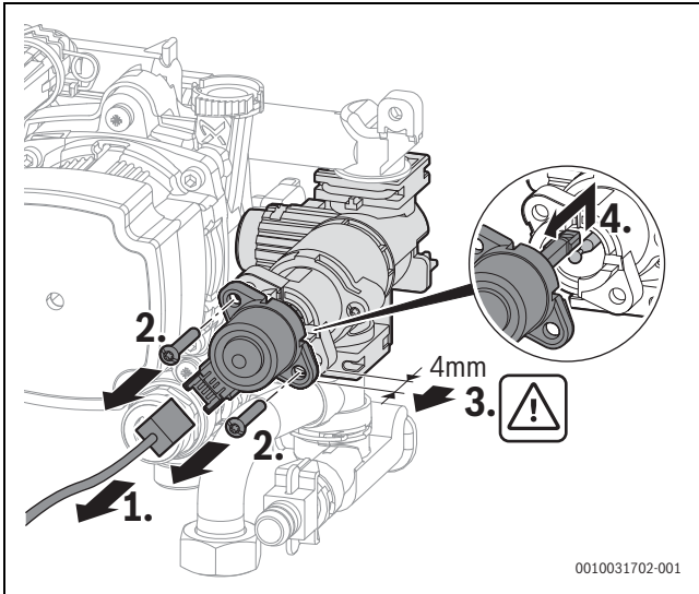
Bild 71 Motor am 3-Wege-Ventil ausbauen (Variante mit Schrauben)
