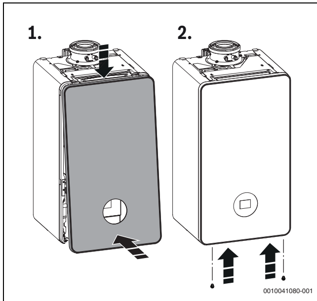
Bild 42 Verkleidung montieren
