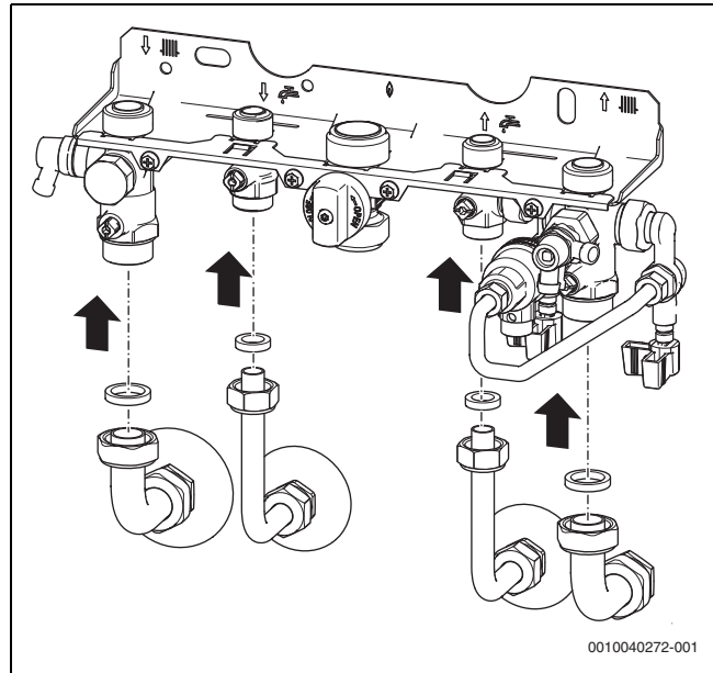
Bild 31 Rohre mit Dichtungen an Montageanschlussplatte (Zubehör) montieren
