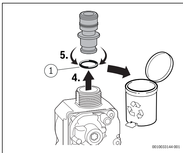
Bild 56 Gassrossel abnehmen
