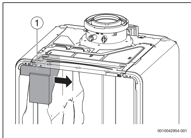
Bild 32 Stützschaum entfernen
