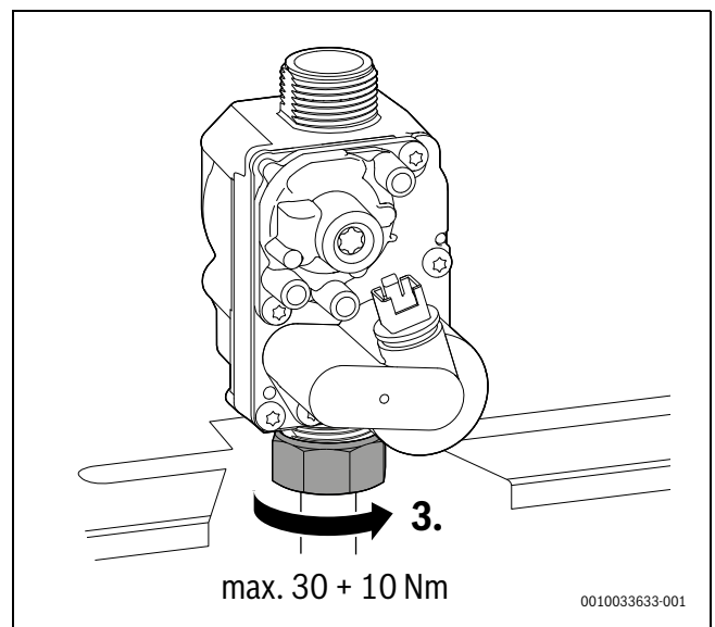
Bild 60 Anzugsdrehmoment beachten
