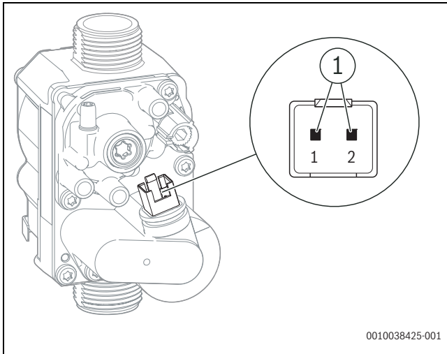
Bild 50 Messstellen an der Gasarmatur
