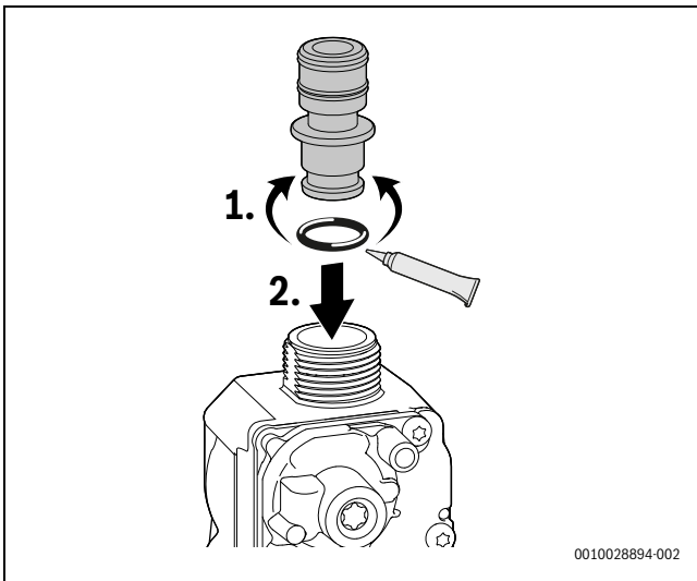
Bild 61 Gassrossel einsetzen
