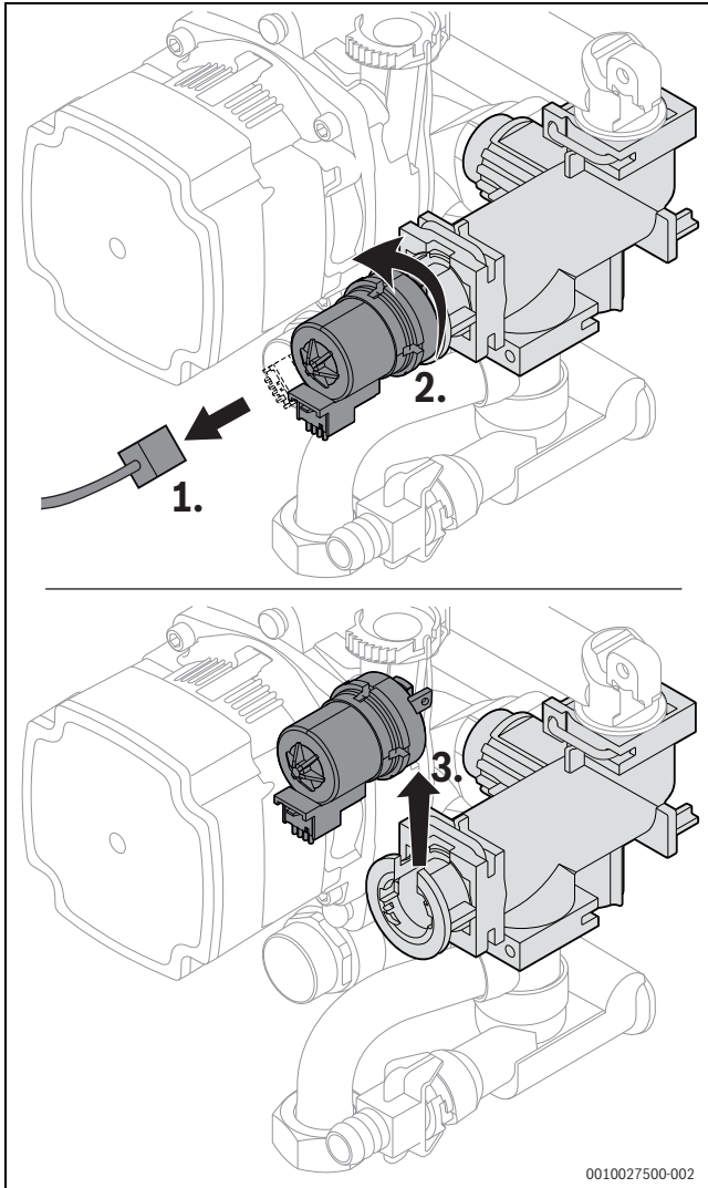
Bild 69 Motor am 3-Wege-Ventil ausbauen (Variante ohne Schrauben)
