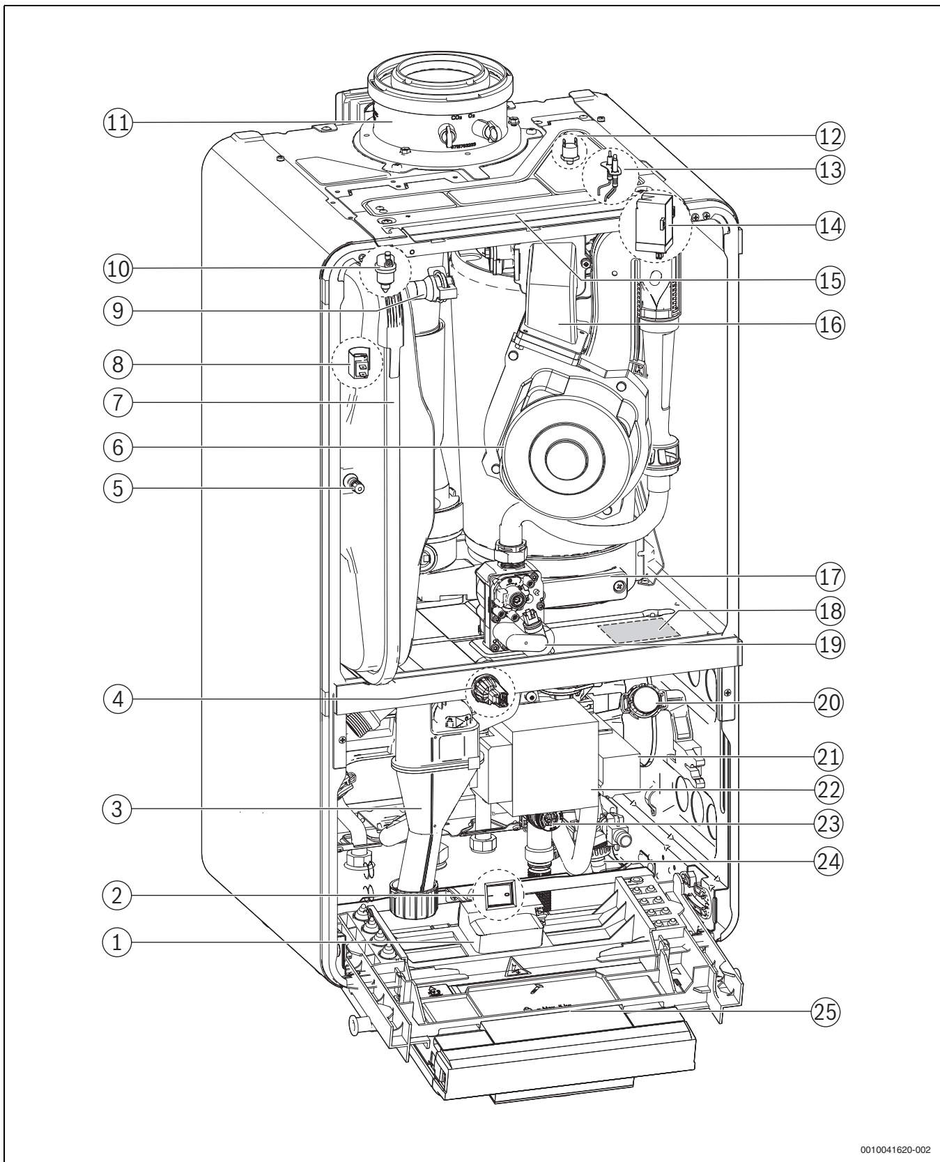
Bild 7 Produktübersicht Speichergerät
