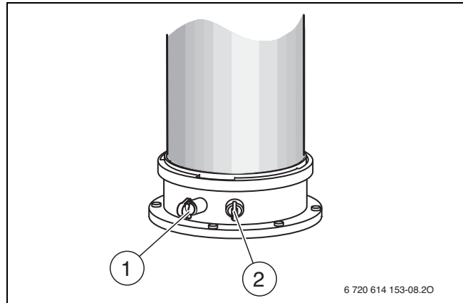
Bild 48 Abgasmessstutzen und Verbrennungsluft-Messstutzen
