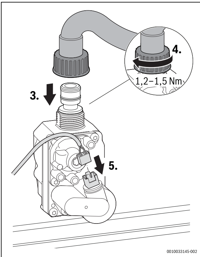
Bild 62 Gasschlauch und Stecker anschließen – Anzugsdrehmoment beachten
