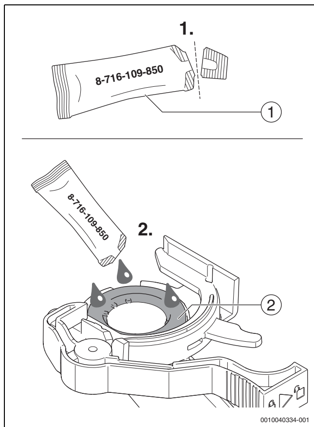
Bild 67 Dichtung fetten
