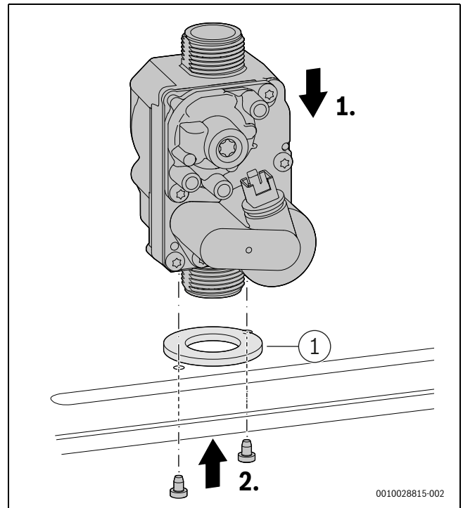
Bild 59 Gasarmatur einbauen
