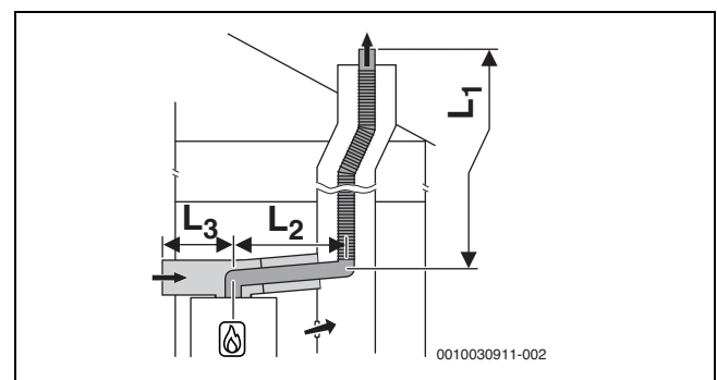
Bild 15 Flexible Abgasführung nach C 53x im Schacht und Luft-Abgas-Führung mit separater Luftzufuhr und konzentrischer Abgasleitung im Aufstellraum
