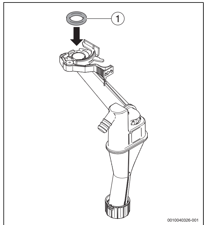
Bild 66 Neue Dichtung am Kondensatsiphon einsetzen
