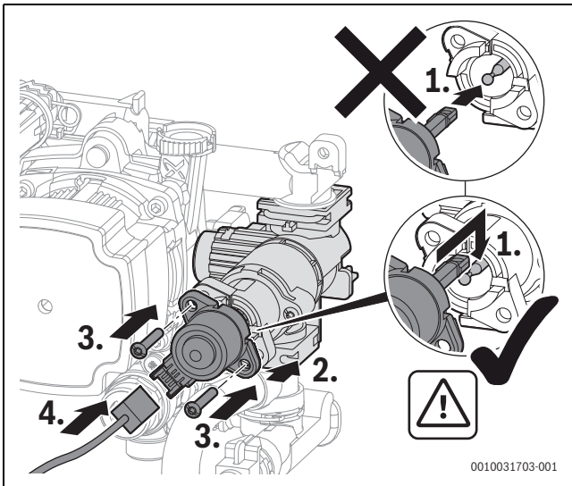
Bild 72 Motor am 3-Wege-Ventil einbauen (Variante mit Schrauben)
