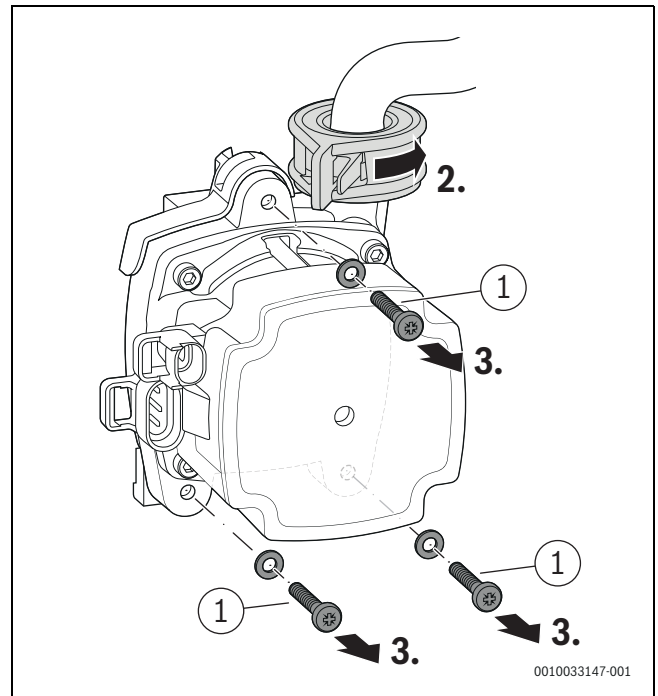
Bild 52 Heizungspumpe entriegeln und Schrauben entfernen
