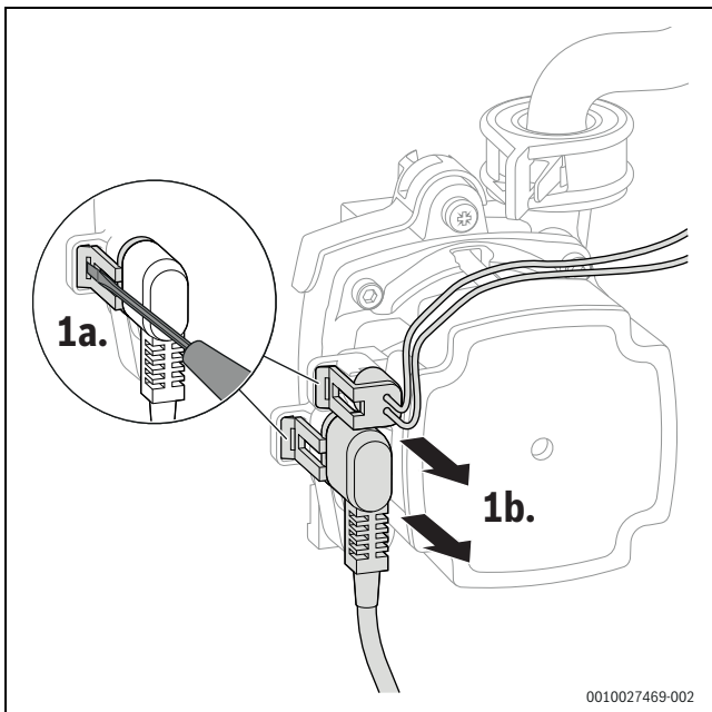
Bild 51 Stecker an der Heizungspumpe abziehen
