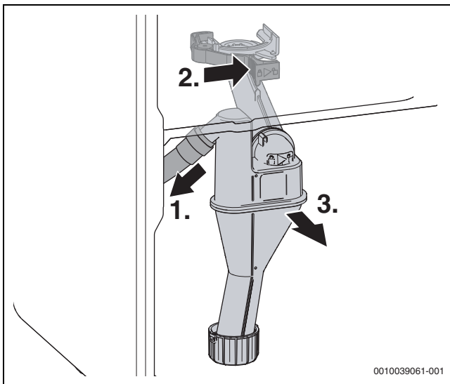
Bild 64 Kondensatsiphon ausbauen
