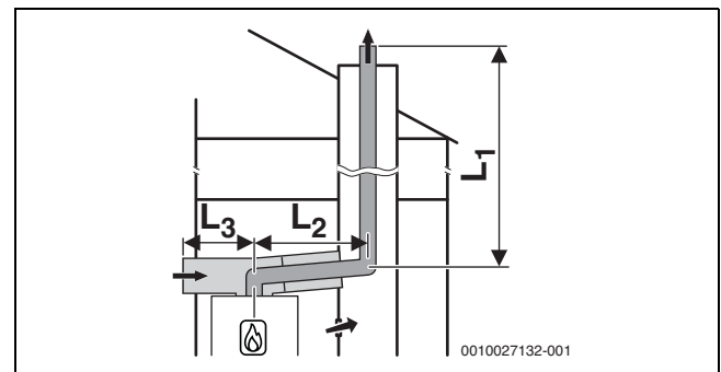
Bild 14 Starre Abgasführung nach C 53x im Schacht und Luft-Abgas-Führung mit separater Luftzufuhr und konzentrischer Abgasleitung im Aufstellraum
