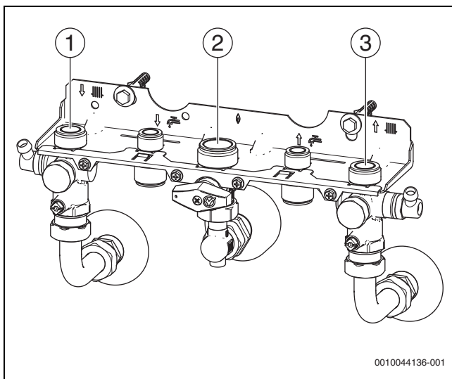
Bild 38 Gas- und wasserseitige Anschlüsse
