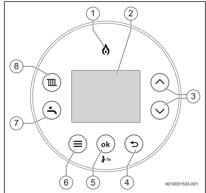
Bild 43 Übersicht
