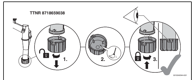
Bild 65 Schmutzfänger reinigen
