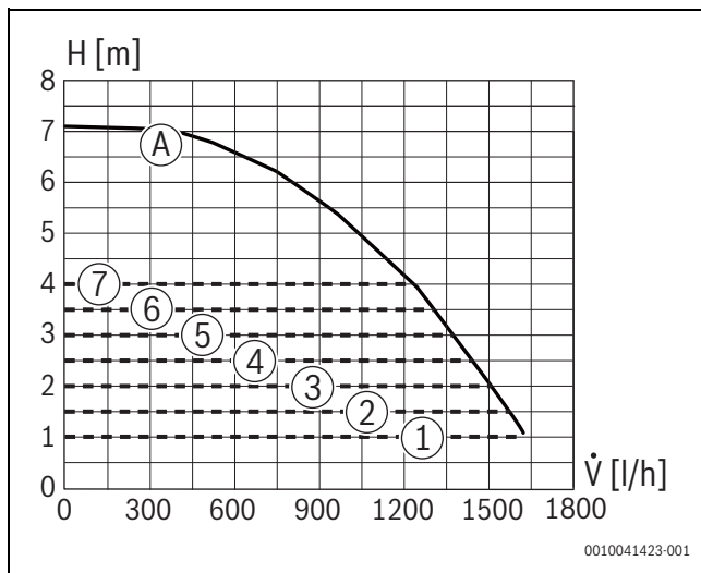
Bild 73 Pumpenkennfelder und Pumpenkennlinien
