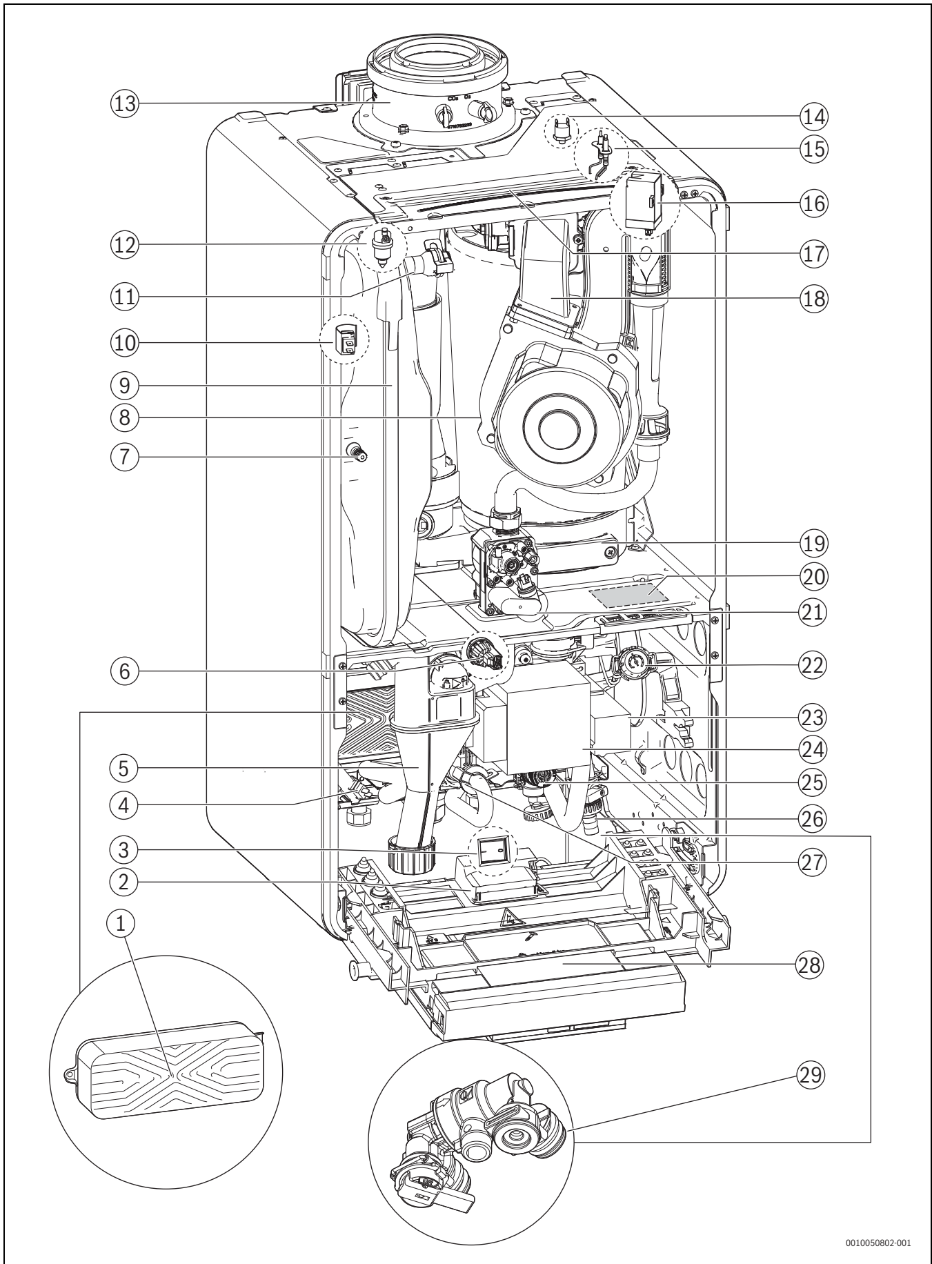
Bild 6 Produktübersicht Kombigerät
