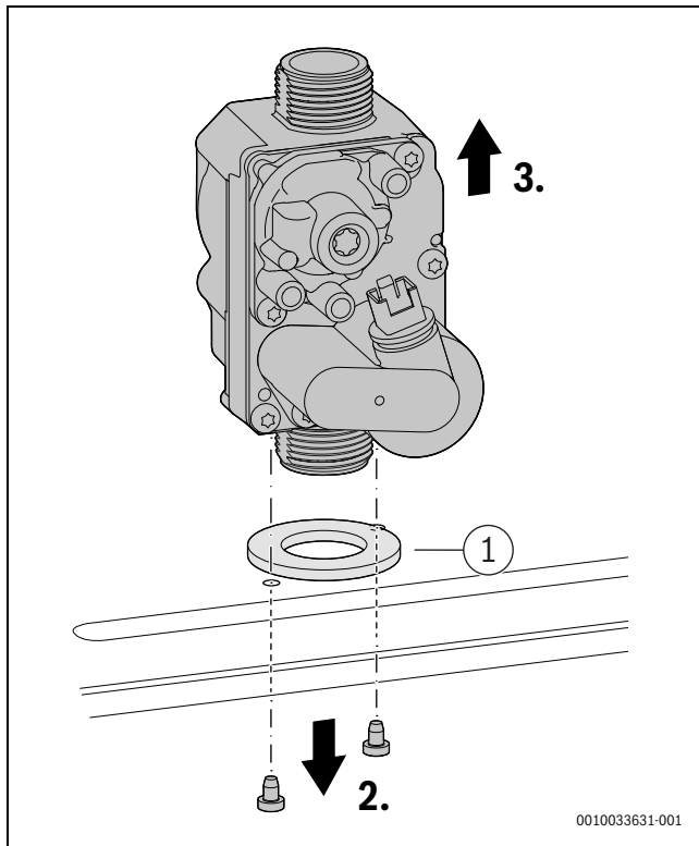
Bild 58 Gasarmatur ausbauen
