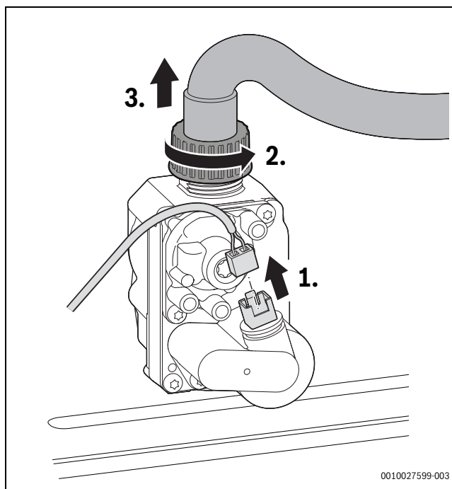
Bild 54 Stecker an der Gasarmatur abziehen und Überwurfmutter mit Gasschlauch abnehmen
