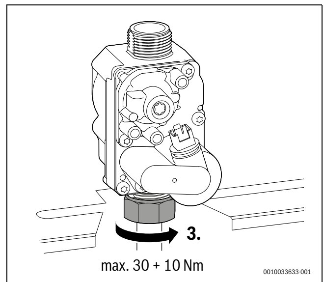
Bild 59 Anzugsdrehmoment beachten
