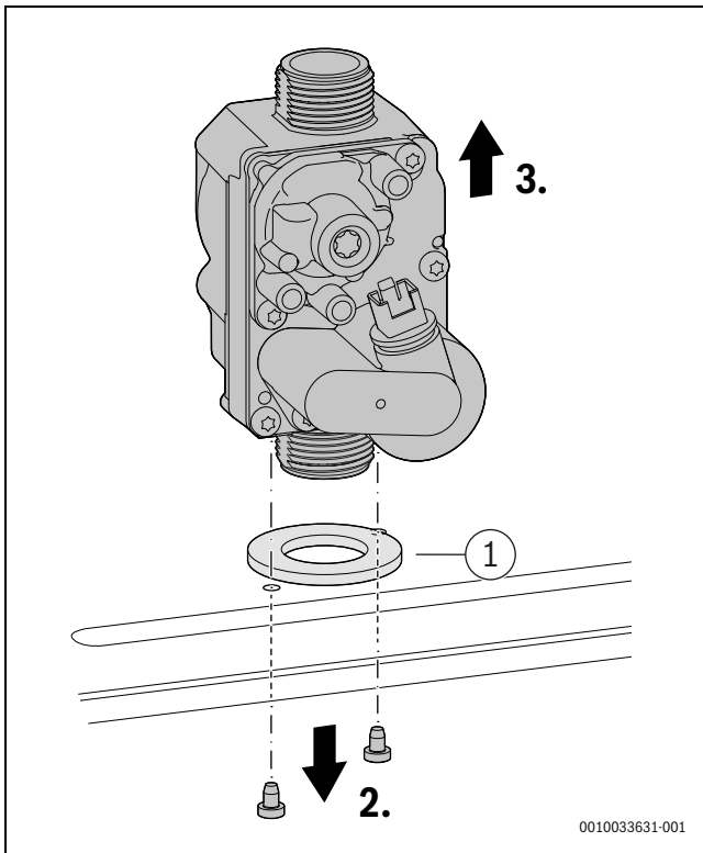
Bild 57 Gasarmatur ausbauen
