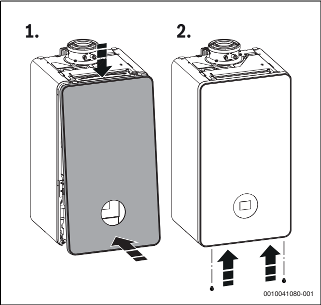
Bild 41 Verkleidung montieren
