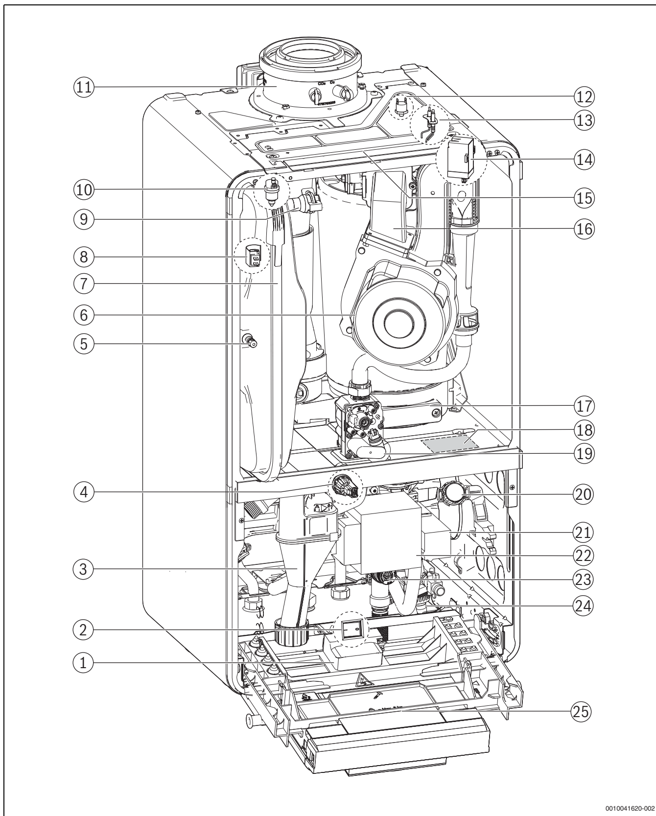
Bild 7 Produktübersicht
