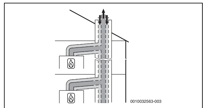
Bild 23 Mehrfachbelegung nach C(10)3x mit konzentrischer Luft-Abgas-Führung im Aufstellraum
