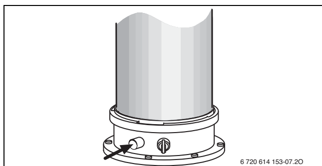
Bild 44 Abgassmessstutzen
