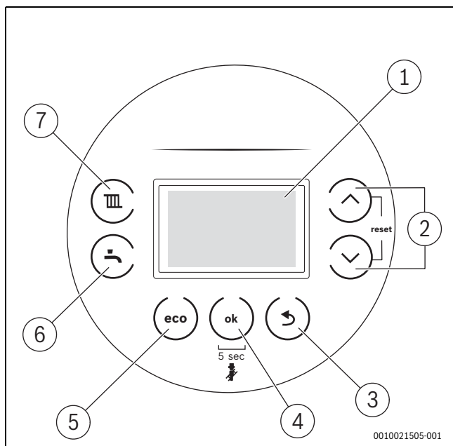
Bild 42 Bedienfeld
