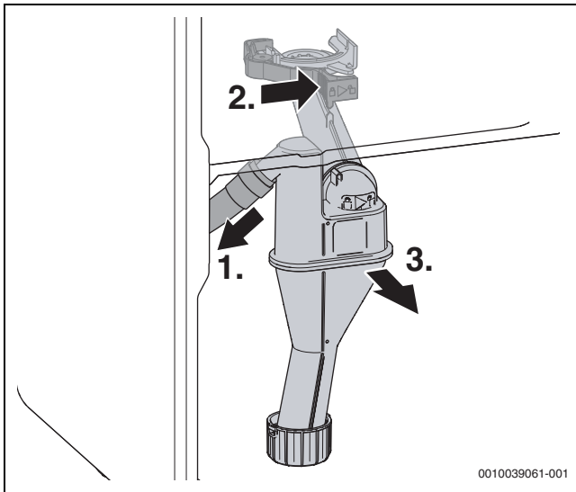
Bild 63 Kondensatsiphon ausbauen
