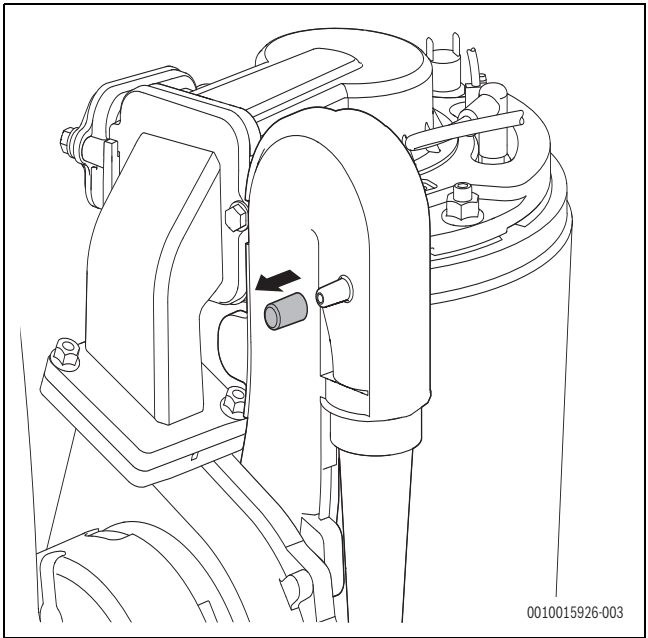
Bild 48 Messstutzen an der Mischeinrichtung
