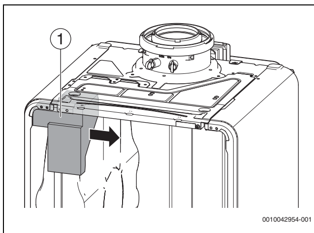
Bild 31 Stützschaum entfernen
