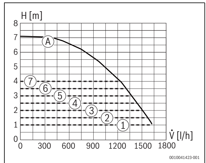
Bild 72 Pumpenkennfelder und Pumpenkennlinien
