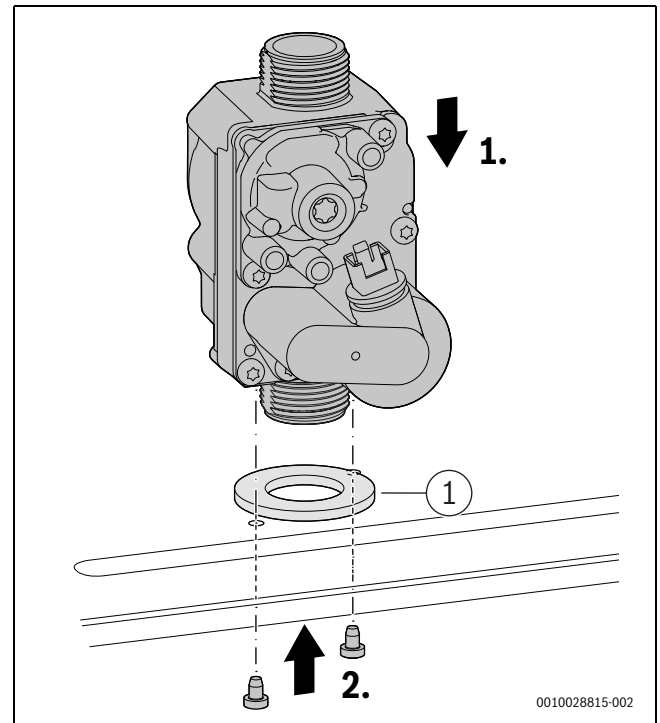
Bild 58 Gasarmatur einbauen
