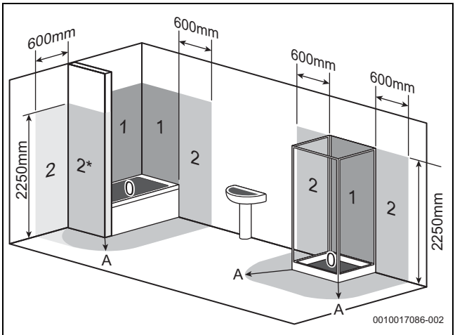
Bild 29 Schutzbereiche (Beispieldarstellung)
