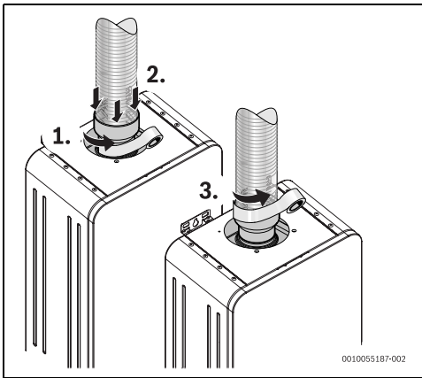
Fig. 22 Installation du type B23
