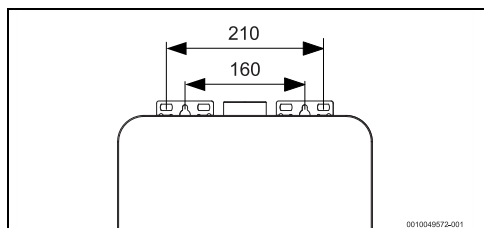
Fig. 19 Points de fixation
