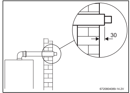
Fig. 23 Dimensions (en mm)
