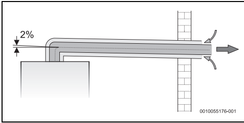
Fig. 21 Installation du type C13
