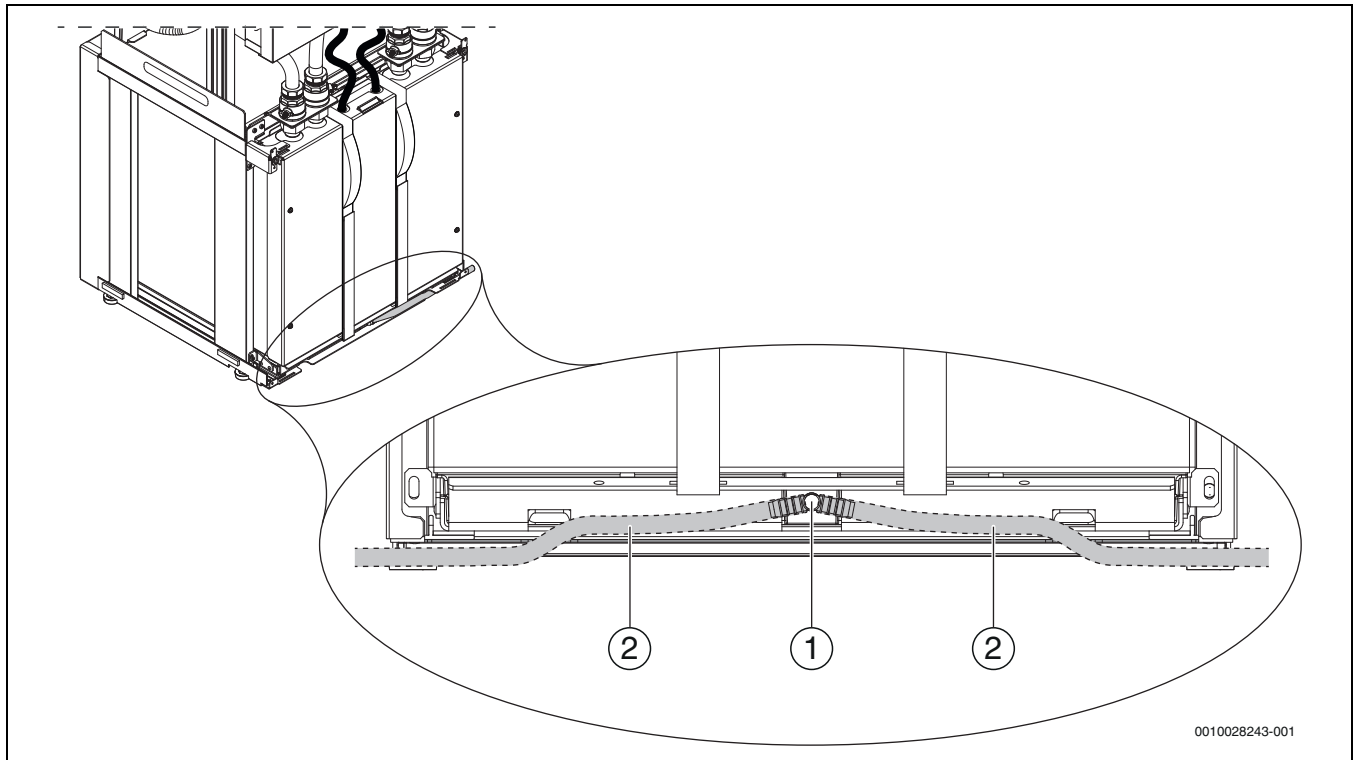
Afb. 13 Aansluiting van de aftapslang
