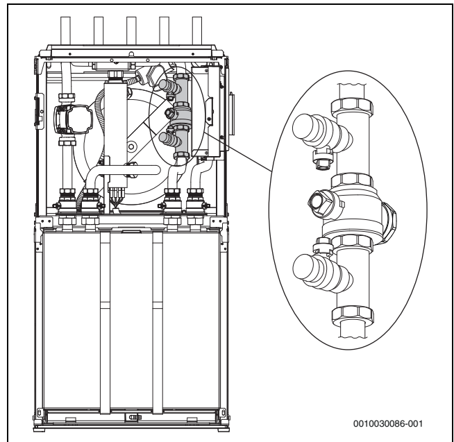
Afb. 27 Vulstelsysteem
