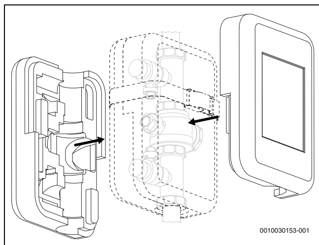
Afb. 34 Isolatie van het vulsysteem
