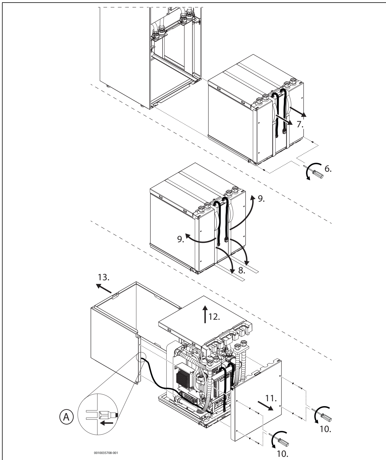
Afb. 40 Bereikbaarheid van het koudecircuit voor omvangrijke installatie- en onderhoudswerkzaamheden, stap 6–13
