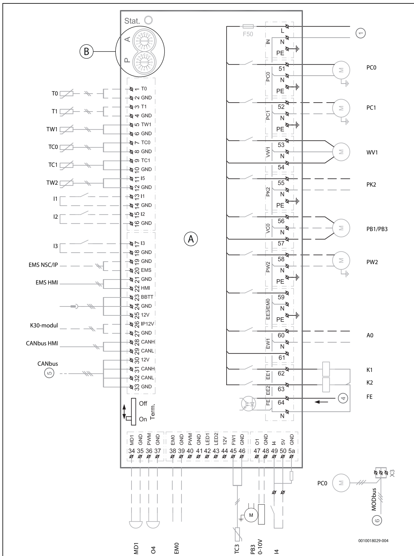
Afb. 52 Schakelschema installatieprintplaat
