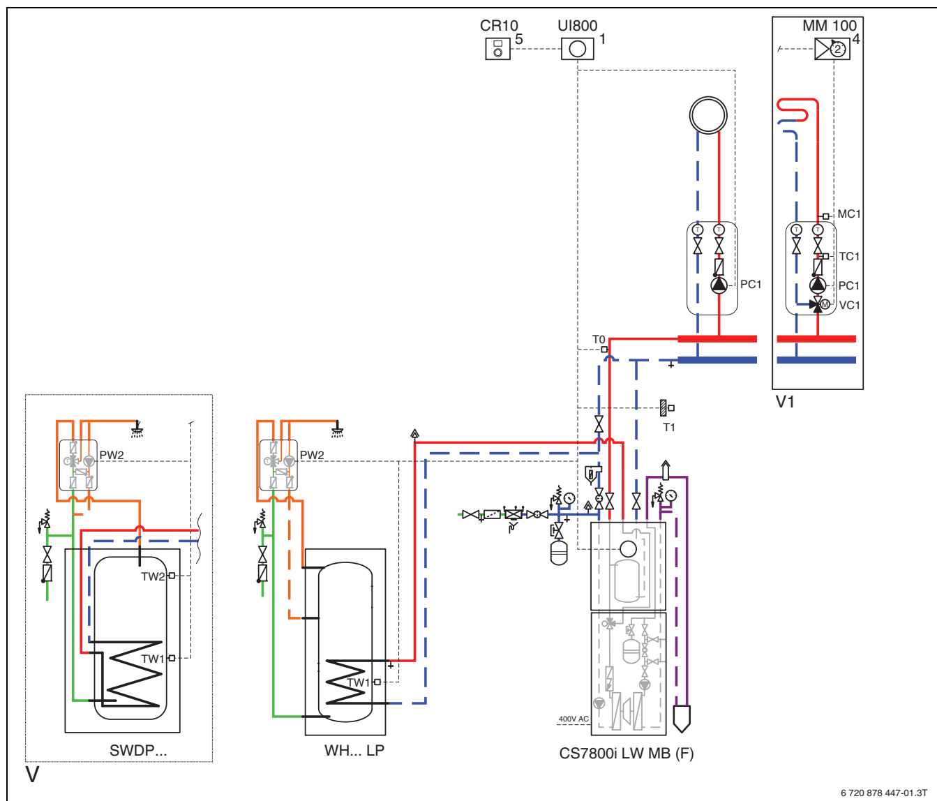
Afb. 46 Buffervat
