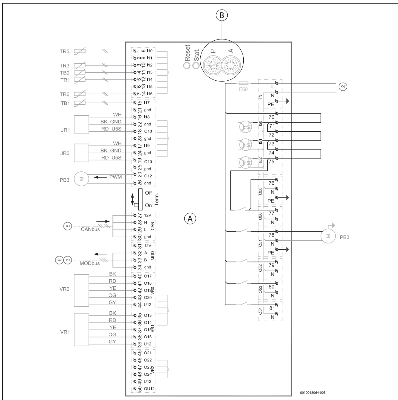
Afb. 53 Schakelschema I/O-module
